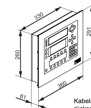
Schaltschrankeinbau (0204)
