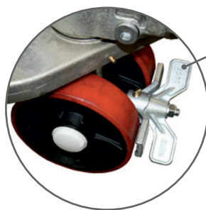
Feststellbremse
