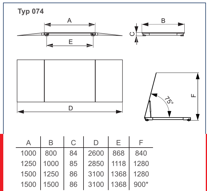
Brückenblechverriegelung
